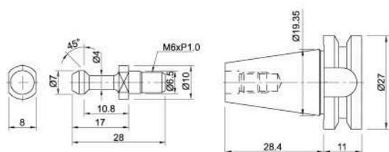
BT15 刀桿錐度尺寸 BT15 SHANK INFORMATION
