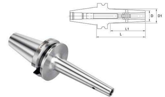
KG(S) 二面接觸細長後拉式高精度銑刀夾頭 DOUBLE FACE CONTACT COLLET CHUCK/KG(S)
