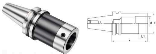
LCK 二面接觸雙刃粗(精)搪刀桿 DOUBLE FACE CONTACT BORING HOLDER/LCK
