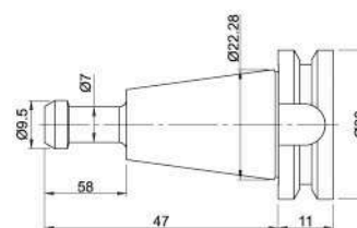
BT20 刀桿錐度尺寸 BT20 SHANK INFORMATION
