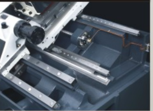
傳動系統
