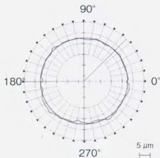
真圓度(同時五軸制御) 〈NAS規格979〉
